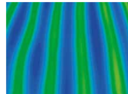
RÖFIX Fliessestrich: Optimale Wärmeabgabe nach 1.5 Stunden (aufgenommen mit Wärmebildkamera)
