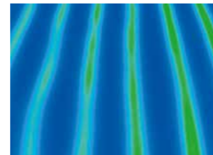
Herkömmlicher Zementestrich: Optimale Wärmeabgabe nach 1.5 Stunden (aufgenommen mit Wärmebildkamera)
